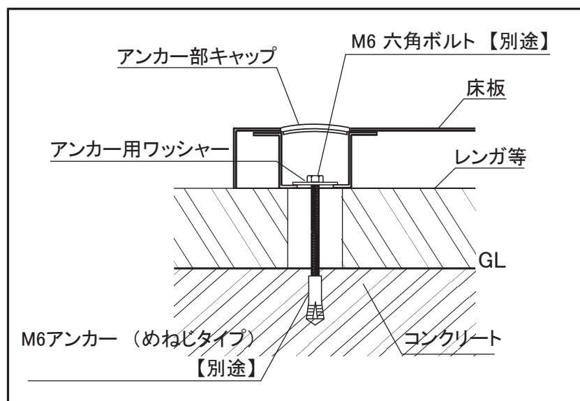
アンカー取付詳細図
